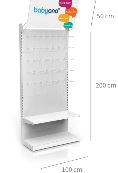
Wide modular display Ekspozytor modułowy szeroki
